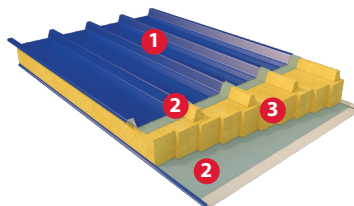
КРОВЕЛЬНАЯ СЭНДВИЧ-ПАНЕЛЬ
