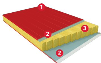
СТЕНОВАЯ СЭНДВИЧ-ПАНЕЛЬ
